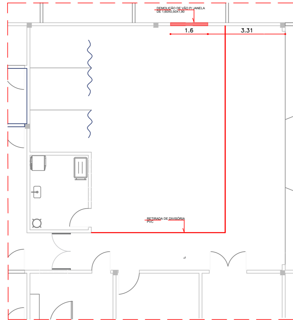
PLANTA BAIXA – DEMOLIÇÃO ESC. 1:100
