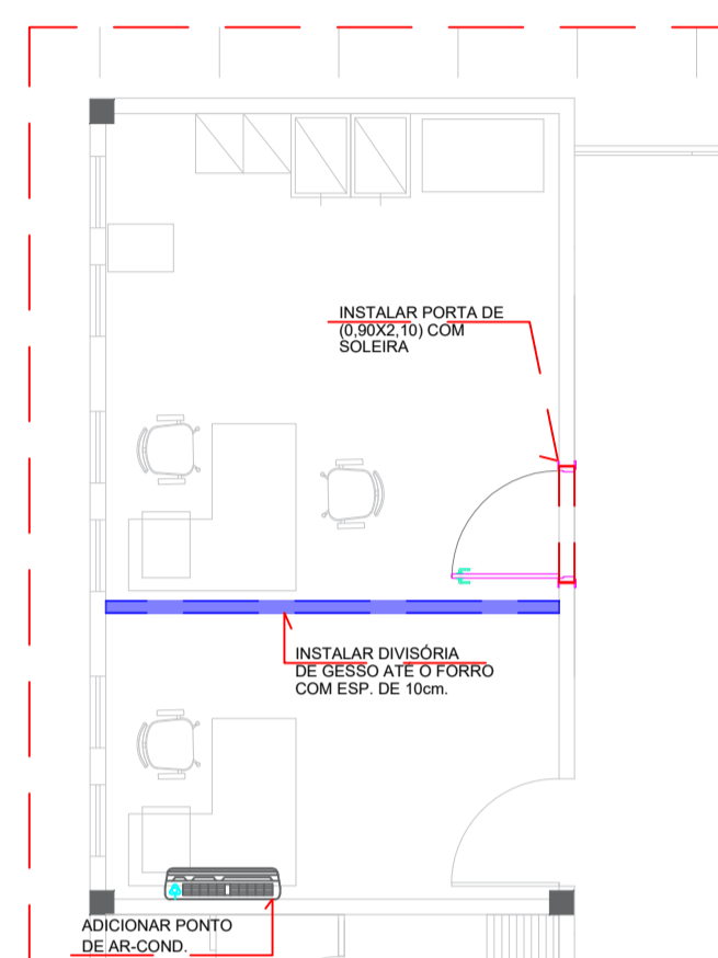
PLANTA BAIXA – CONSTRUÇÃO ESC. 1:100
