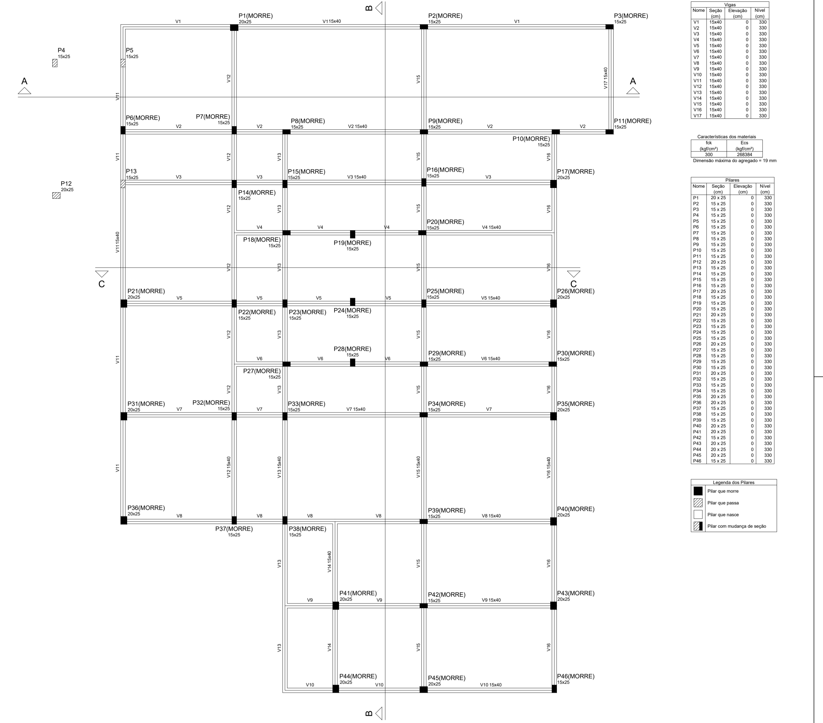
Forma do pavimento +3.30 (Nível 330) escala 1:50
