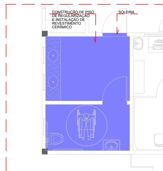
PLANTA BAIXA – CONSTRUÇÃO ESC. 1:100
