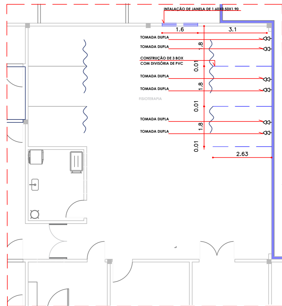
PLANTA BAIXA – CONSTRUÇÃO/PONTOS ESC. 1:100
