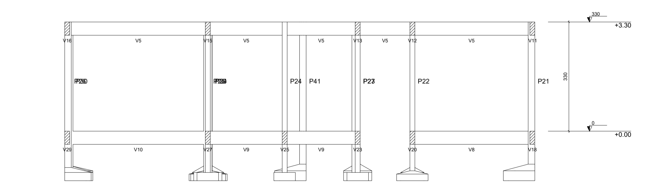
Corte C-C escala 1:50
