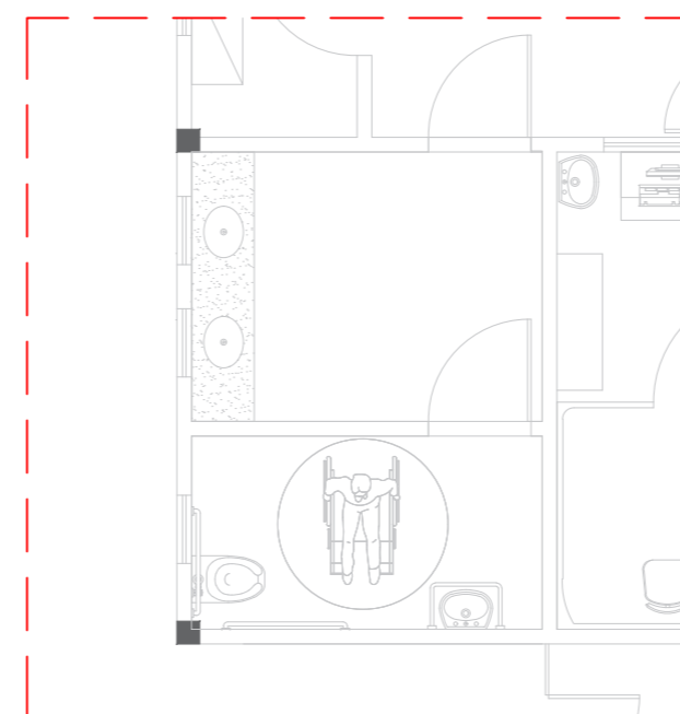
PLANTA BAIXA – PREVISTA ESC. 1:100
