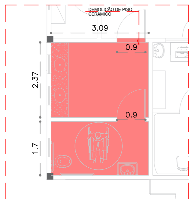
PLANTA BAIXA – DEMOLIÇÃO ESC. 1:100
