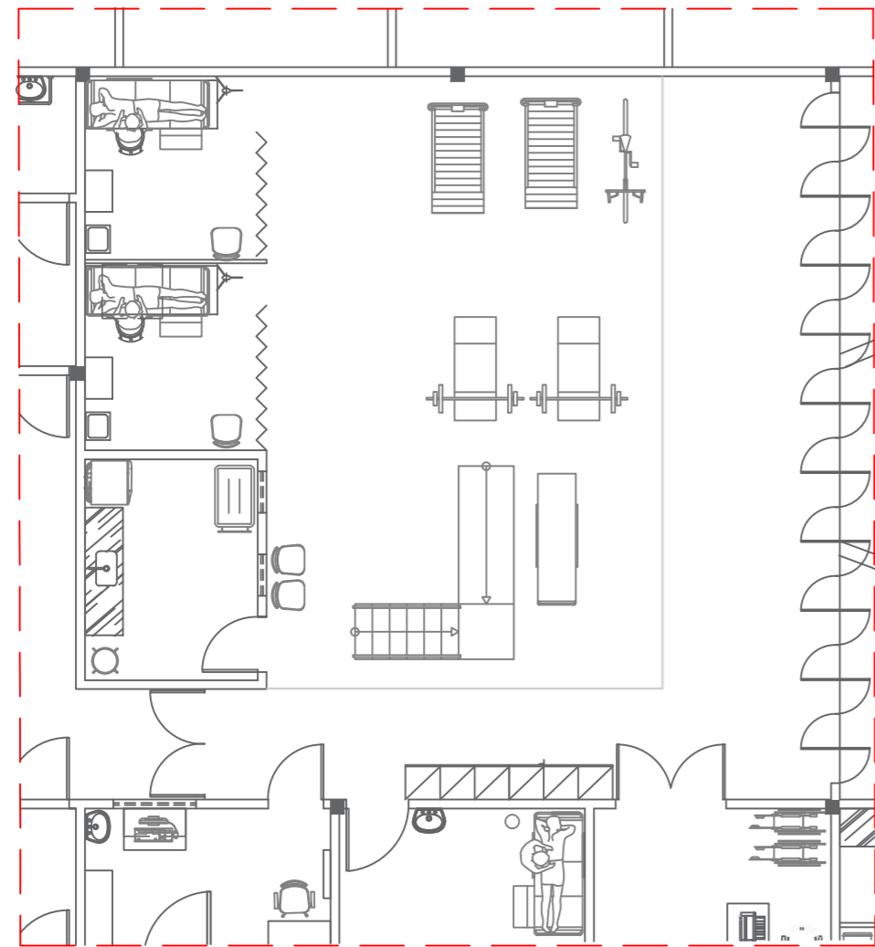
PLANTA BAIXA – EXISTENTE ESC. 1:100
