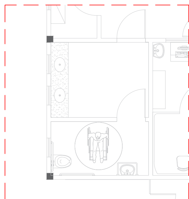
PLANTA BAIXA – EXISTENTE ESC. 1:100
