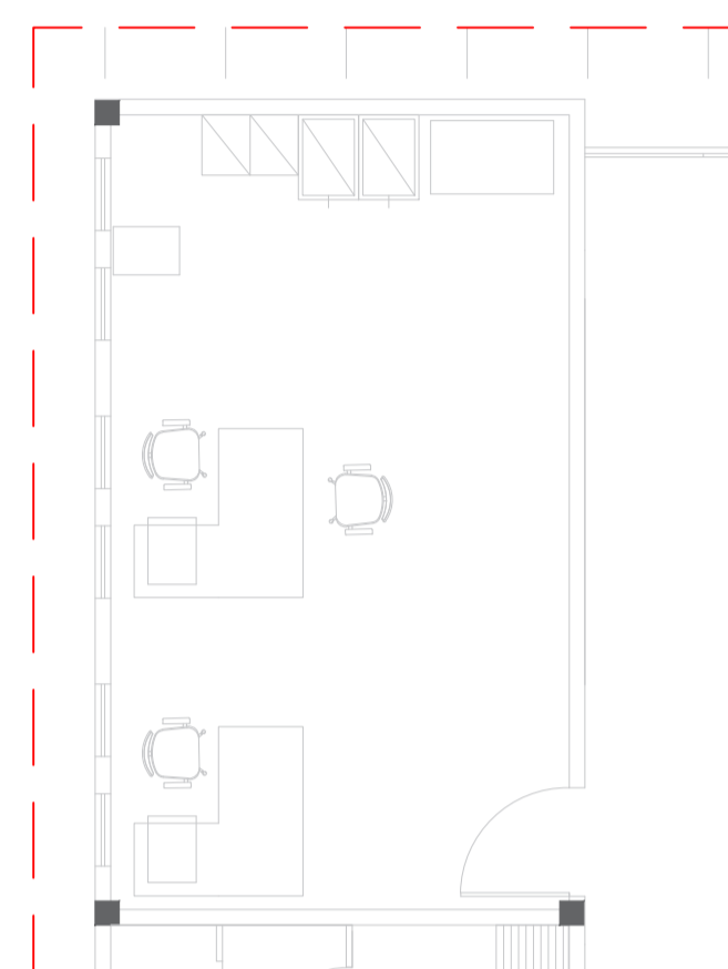
PLANTA BAIXA – EXISTENTE ESC. 1:100
