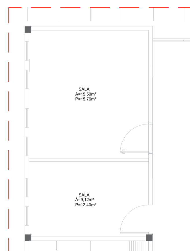
PLANTA BAIXA – PREVISTA ESC. 1:100
