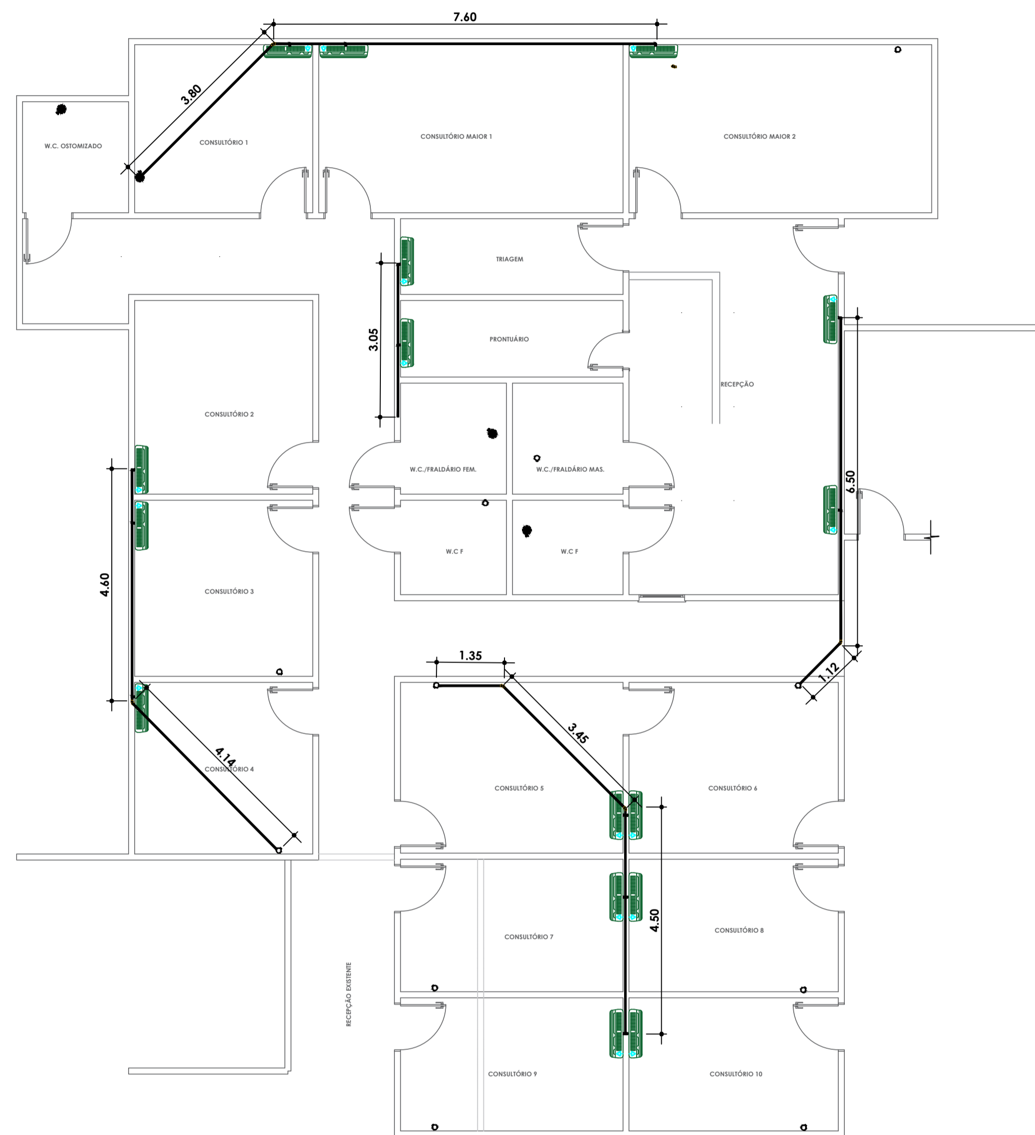
PLANTA BAIXA CLIMATIZAÇÃO – DRENO ESC. 1:50
